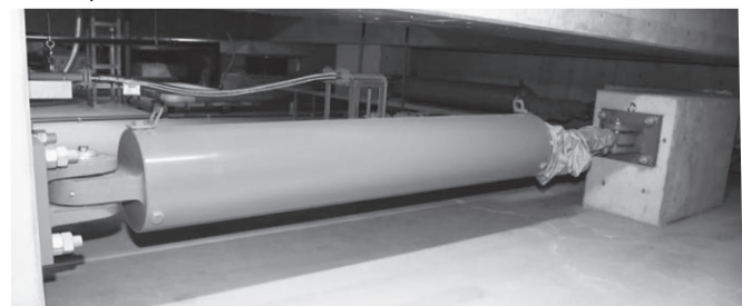
▲市役所本庁舎に設置されている免震オイルダンパー（12基全ての検査データが改ざん、そのうち2基が顧客契約基準を満たしていないことが発覚）
